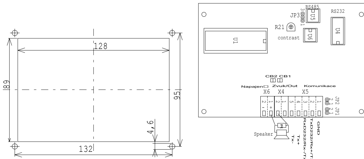
Obr. 2 Montážní rozměry a rozmístění propojek a konektorů.
