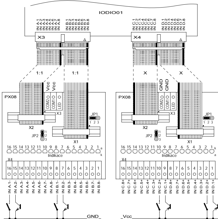
Zapojení vstupů se společným mínus (kontakt a snímač s tranzistorem npn)
